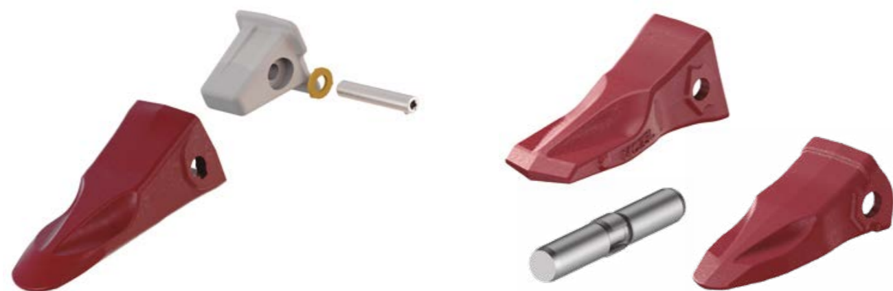
СИСТЕМА С БОКОВЫМ ПАЛЬЦЕМ И БЕЗУДАРНЫМ КРЕПЛЕНИЕМ ДЛЯ АДАПТЕРОВ CATERPILLAR*
